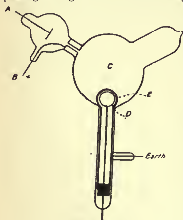
Electrometer FIG. 24.
